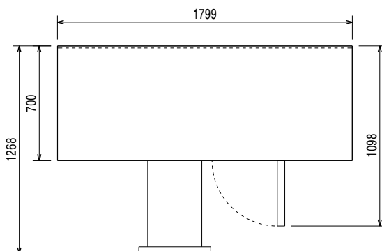
Boven aanzicht
